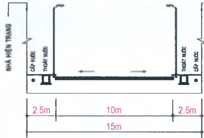
MẶT CẮT 2-2 (ĐƯỜNG LƯƠNG VĂN CÙ)
