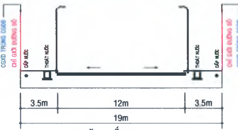
MẶT CẮT 1-1 (ĐƯỜNG NGÔ GIA TỰ)
