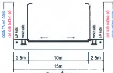
MẶT CẮT 2-2 (ĐƯỜNG LƯƠNG VĂN CÙ)
