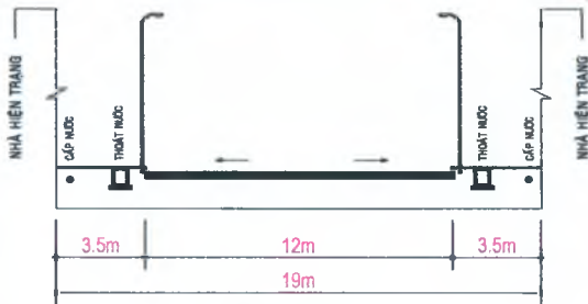
MẶT CẮT 1-1 (ĐƯỜNG NGÔ GIA TỰ)
