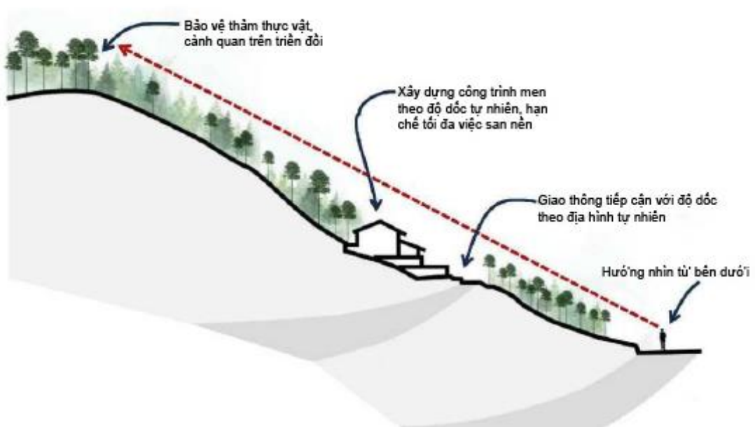
Hình 1 Minh họa phương án được khuyến khích khi xây dựng công trình trên địa hình đồi dốc.
