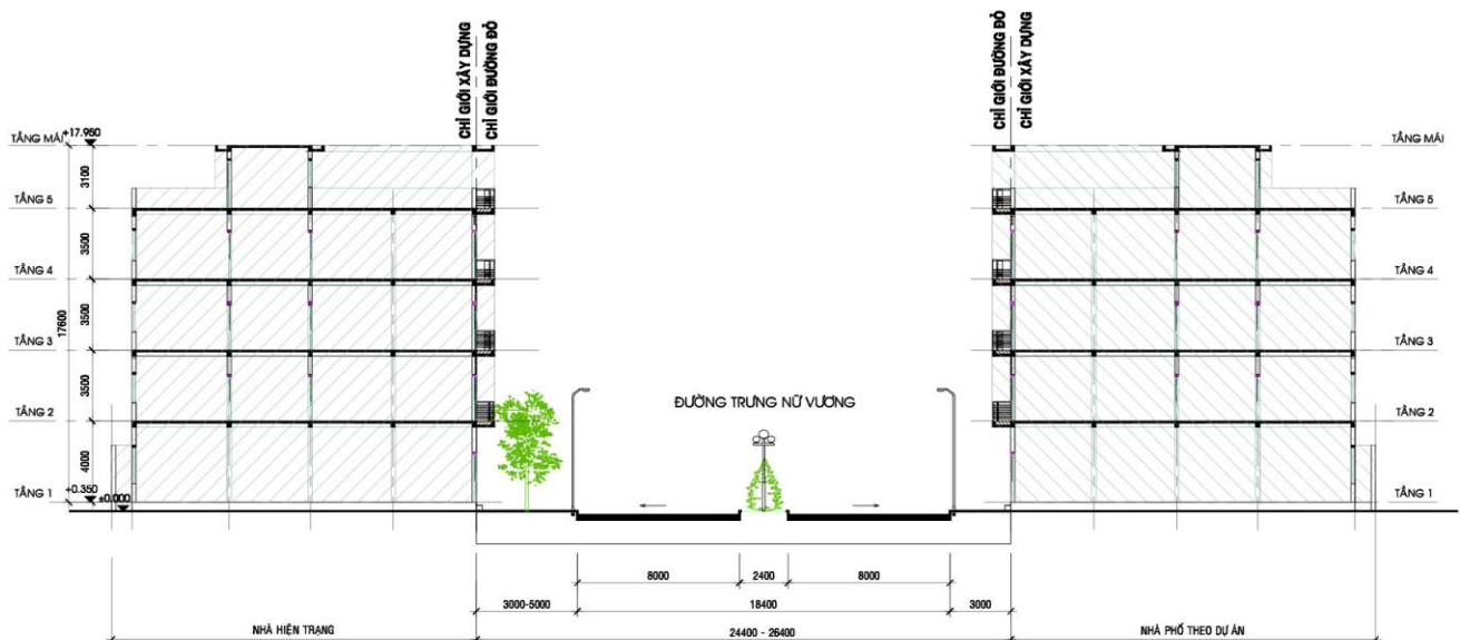
MẶT CẮT 12 - 12 (CẮT NGANG ĐƯỜNG TRƯNG NỮ VƯƠNG)
